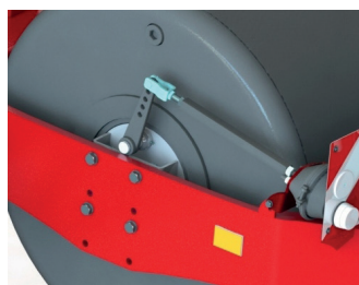
SVAHOVÁ BRZDA bubnová brzda prostředního válce
