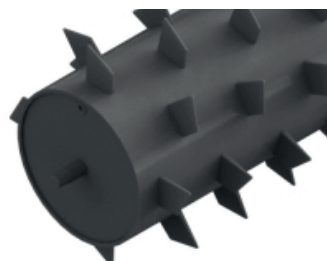
VÁLEC AERÁTOR GOLEM 540: ø válce 720 mm GOLEM 300: ø válce 1020 mm síla stěny 20 mm
