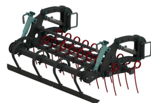
SMYKOVÁ LIŠTA (L-PROFIL) a dvouřadé prutové brány
